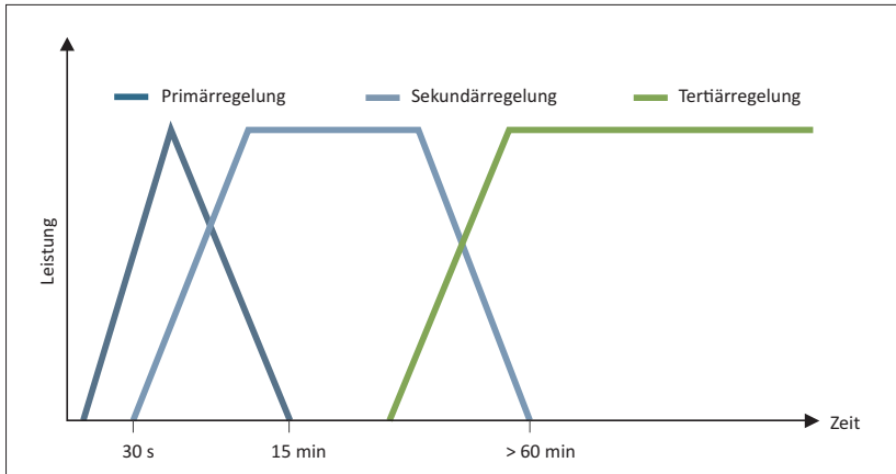
Abb. 3.3.3.2.4: Aufbau der drei Regenelemente – Im Primärregelmarkt müssen Anbieter innerhalb von 30 s positive oder negative Regelleistung zur Verfügung stellen und maximal 15 min erbringen. | Quelle: Younicos | Abb. RENAC
