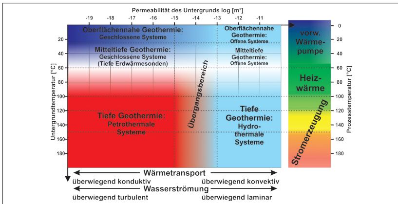
Abb. 3.1.7.2: Definitionsmöglichkeiten für geothermische Nutzsysteeme in Abhängigkeit von der Lagerstätten-Permeabilität und der Erschließungstiefe | Quelle: Sass 2012
