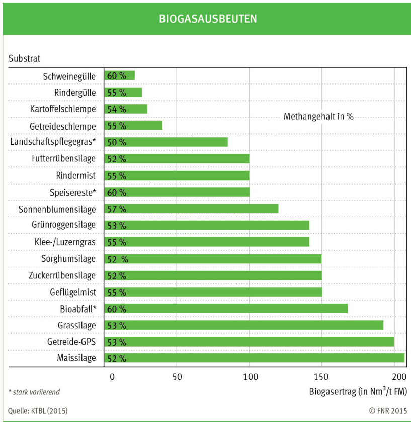
Abb. 3.1.5.2: Biogasausbeuten nach Substrat in Nm 3 /t FM) Quelle: FNR 2015; KTBL 2015
