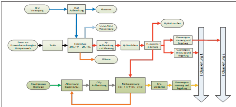
Abbildung 4.14 Blockflussbild einer Power-to-Gas Anlage mit Methanisierung 26
