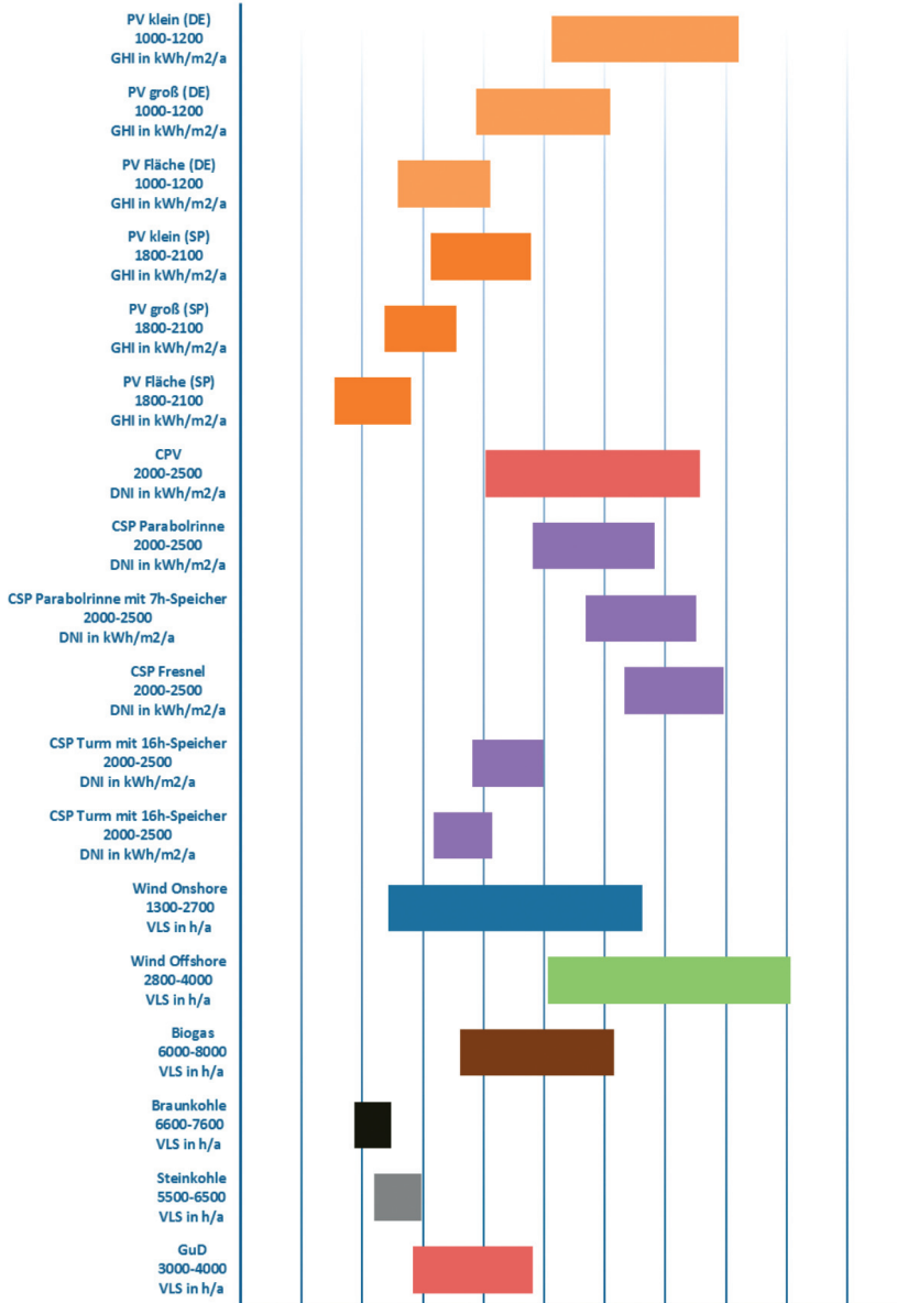
Abb. 6.1.2: Die Zahlen unter der jeweiligen Technologie geben die jährlich geleisteten Volllaststunden an – bei Solaranlagen ist es die Stromausbeute pro Quadratmeter / Quelle: Fraunhofer ISE
