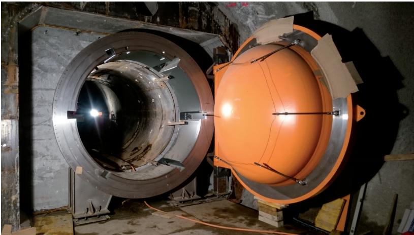
Abb. 3.3.1.3.3: Felskaverne als Druckbehälter | Quelle: zVg
