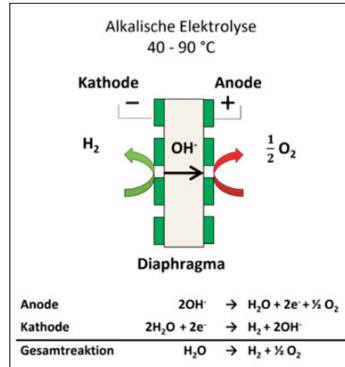
Abbildung 4.4: Alkalische Elektrolyse [DLR- Wasserstoff als Fundament der Energiewende]
