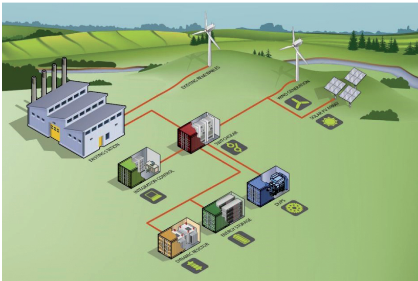
Abb. 3.1.9.1.1 Dezentrales Wind oder Solarstrom Hybridssystem | Quelle: Hydro Tasmania
