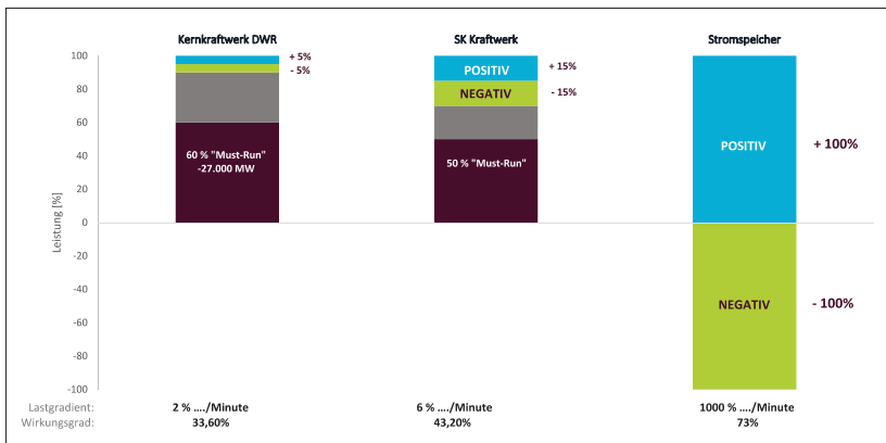
Abb. 3.3.3.2.1: Speicher sind der Schlüssel dazu, das alte Energiesystem in dem Maße zu schrumpfen wie das neue wächst. Vor allem Batterien sind mit Abstand die effizienteste Lösung um Flexibilität in unsere Netze zu bekommen: Sie können 100% ihrer Leistung zur Verfügung stellen und reagieren um Größenordnungen schneller – weshalb insgesamt weniger Regelleistung benötigt wird
