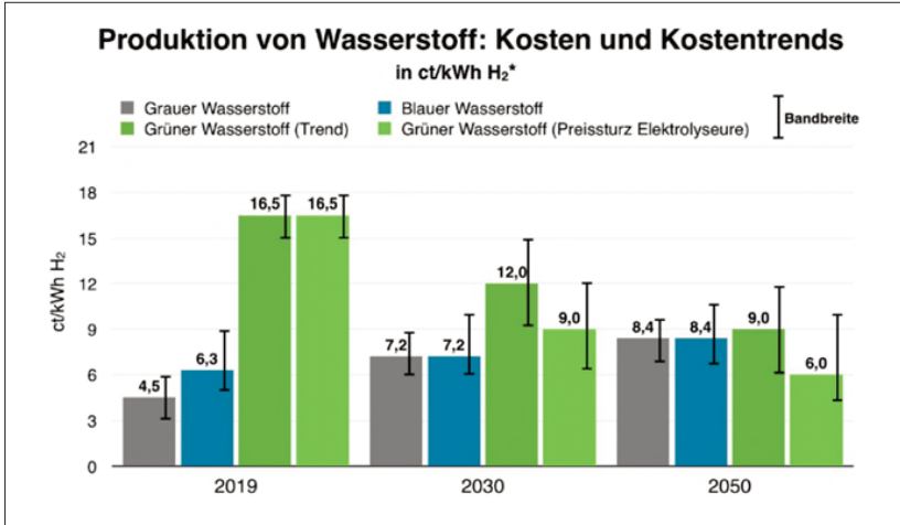
Abbildung 4.17: Gegenwärtige und zukünftige erwartete Wasserstoffherstellungskosten in Westeuropa 31
